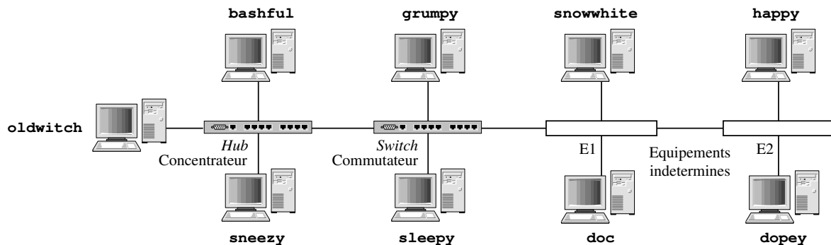
FIGURE 1 – Architecture d'un réseau.
